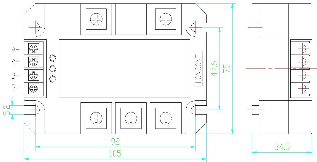
外形尺寸 105*75*35 mm
