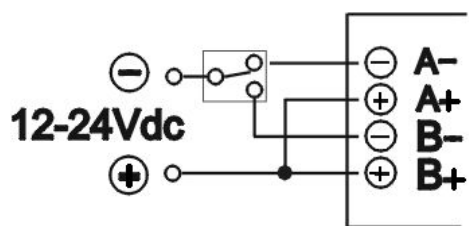
正反输入控制端共阳接法
