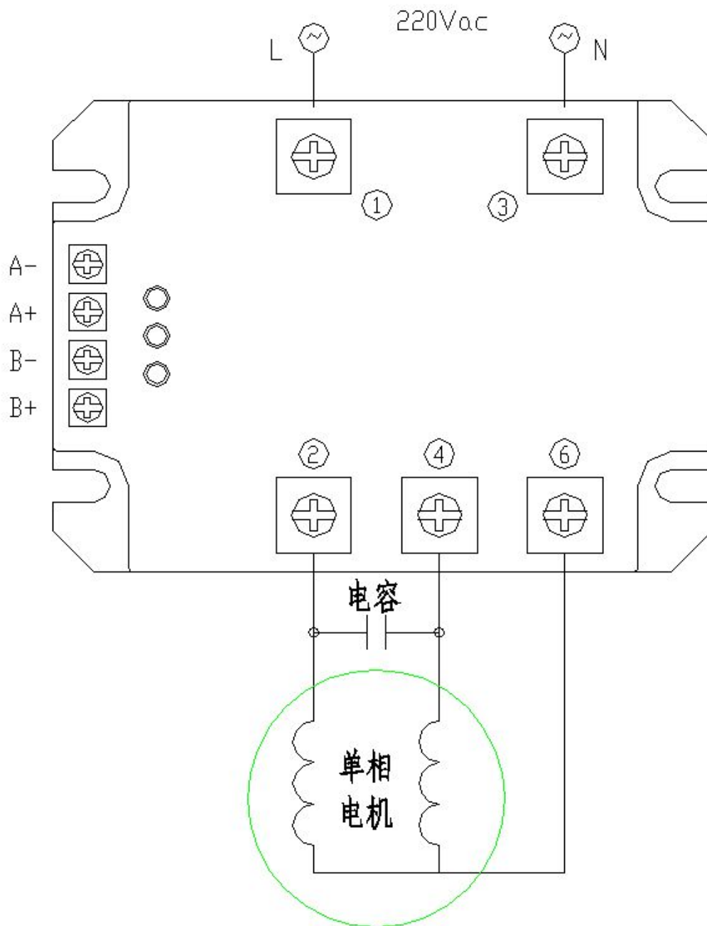
接线图，其中①和③脚为交流电源输入，②④⑥脚接负载。
