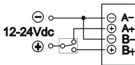
正反输入控制端共阴接法
